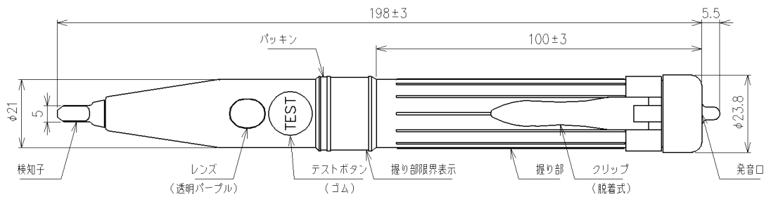
外形寸法図 [mm]
