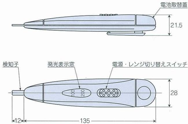
低圧用検電器 MODEL DX-04 (単位mm)
