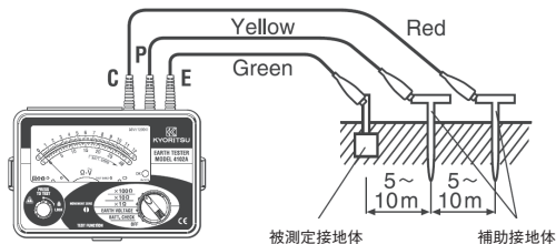
M-4102Aを使用した測定例
