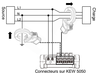
Monophasé à 3 fils
