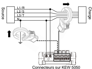
Triphasés à 4 fils
