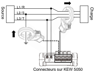
Triphasés à 3 fils
