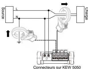
Monophasé à 2 fils
