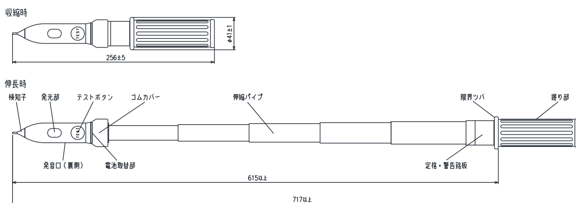
外形寸法図 [mm]
